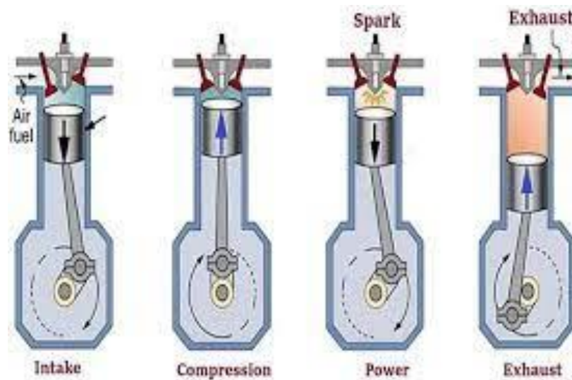
往返活塞推動示意圖
