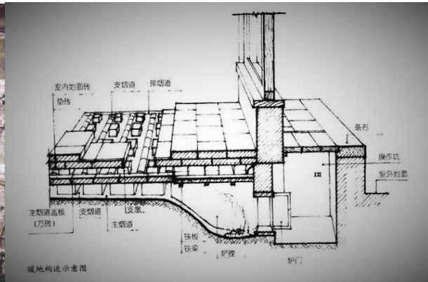
圓明園地暖遺迹實景(左)及地暖構造示意圖(右)
