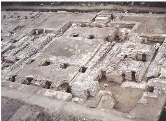
圓明園地暖遺迹實景(左)及地暖構造示意圖(右)
